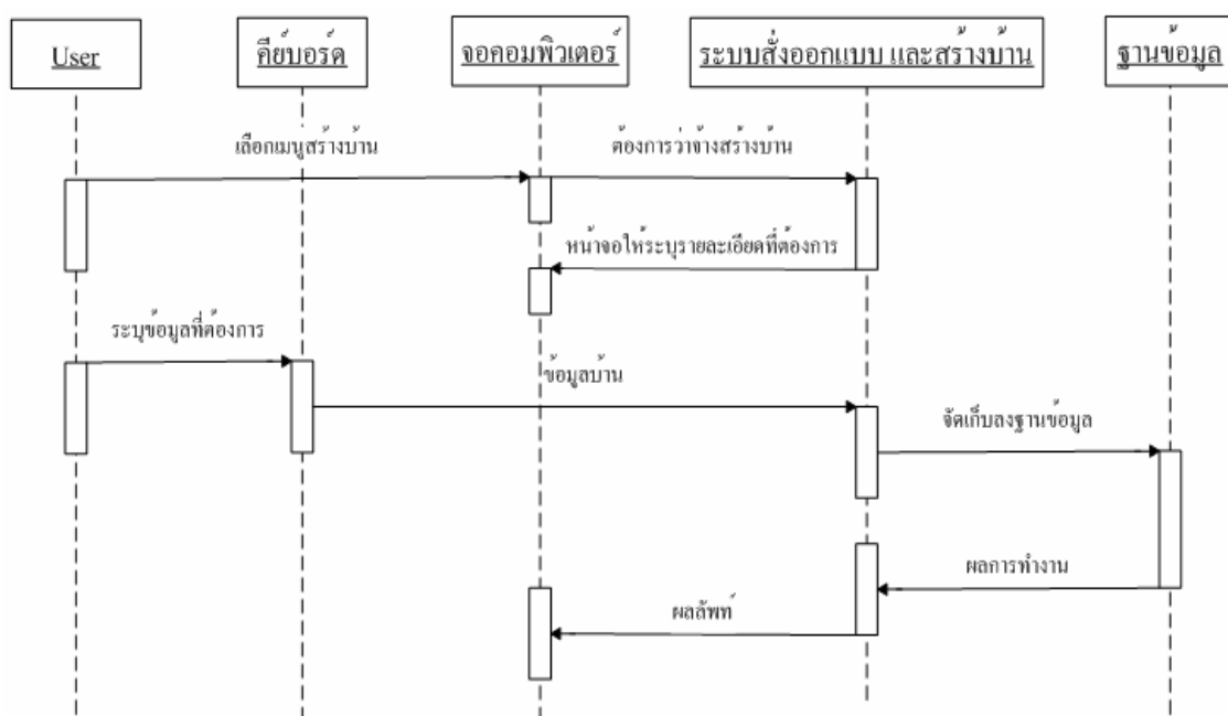
รูปที่ 9-9 ขั้นตอน ของการว่าจ้างสร้างบ้าน
