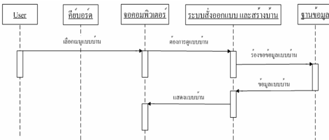
รูปที่ 9-6 ขั้นตอน ของการเข้าดูแบบบ้าน
