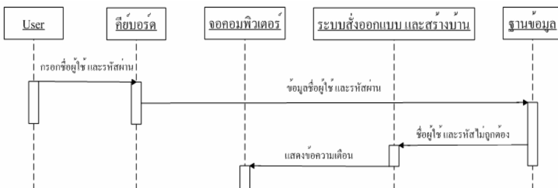
รูปที่ 9-5 ขั้นตอน ของการ Sign in กรณีข้อมูลไม่ถูกต้อง
