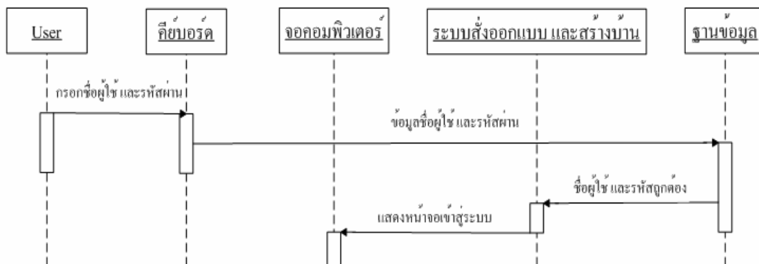
รูปที่ 9-4 ขั้นตอน ของการ Sign in กรณีข้อมูลถูกต้อง
