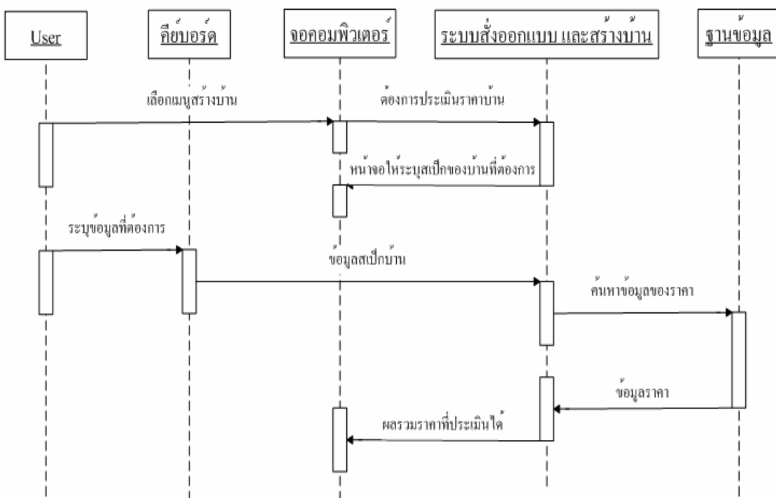
รูปที่ 9-10 ขั้นตอน ของการประเมินราคาบ้าน
