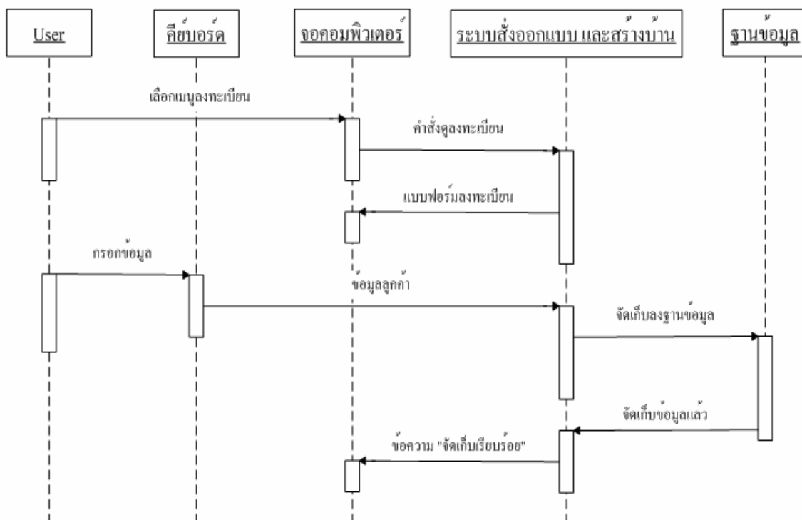
รูปที่ 9-2 ขั้นตอน ของการลงทะเบียนกรณีข้อมูลถูกต้อง
