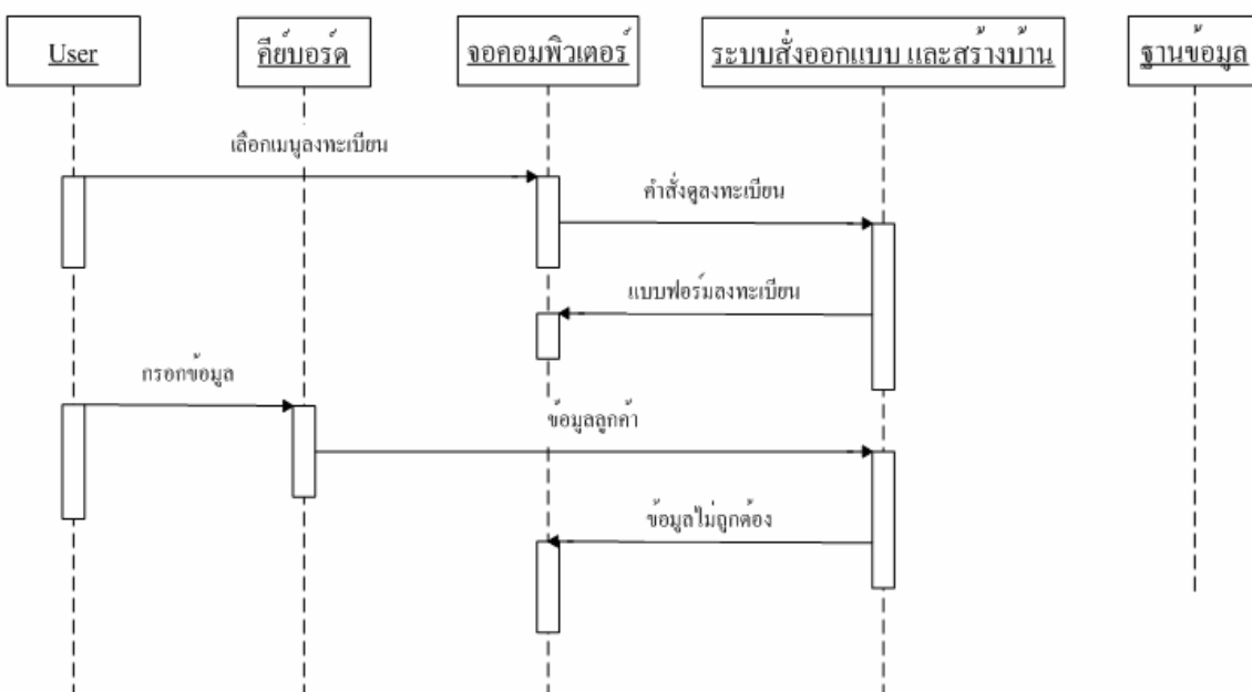
รูปที่ 9-3 ขั้นตอน ของการลงทะเบียนกรณีข้อมูลไม่ถูกต้อง
