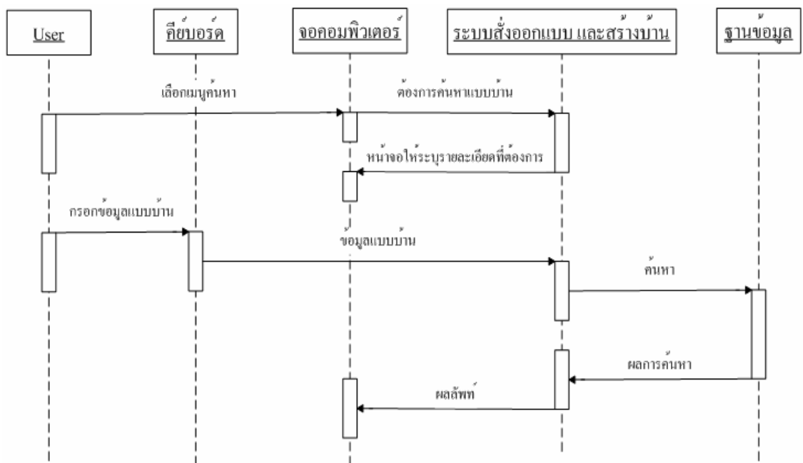
รูปที่ 9-7 ขั้นตอน ของการค้นหาแบบบ้าน
