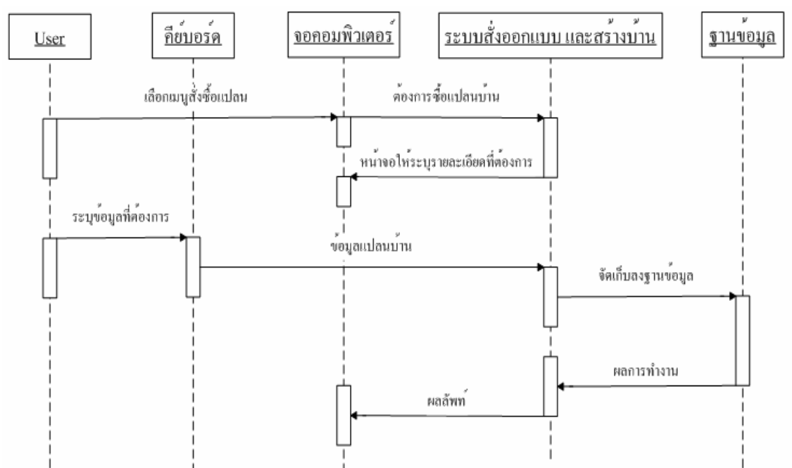
รูปที่ 9-8 ขั้นตอน ของการสั่งซื้อแบบบ้าน
